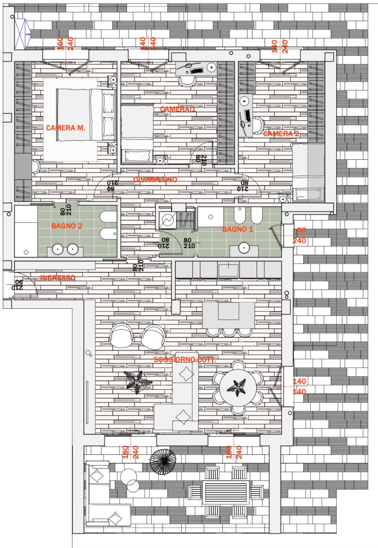
APPARTAMENTO 1 - PIANO TERRA - SCALA 1:50
