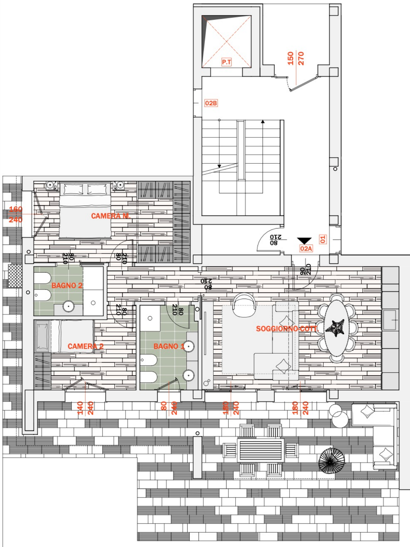
APPARTAMENTO 2A - PIANO TERRA - SCALA 1:50
